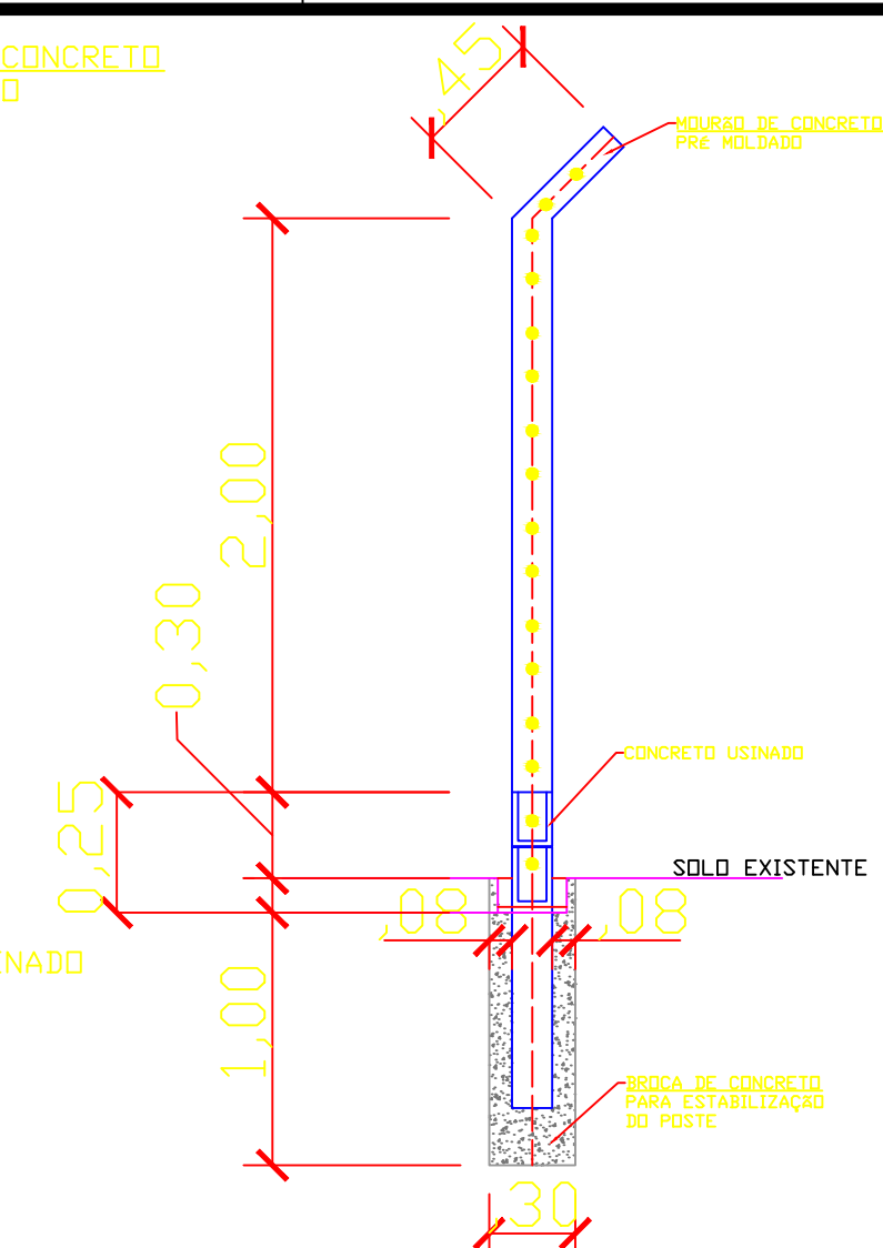
CORTE ESQUEMÁTICO
