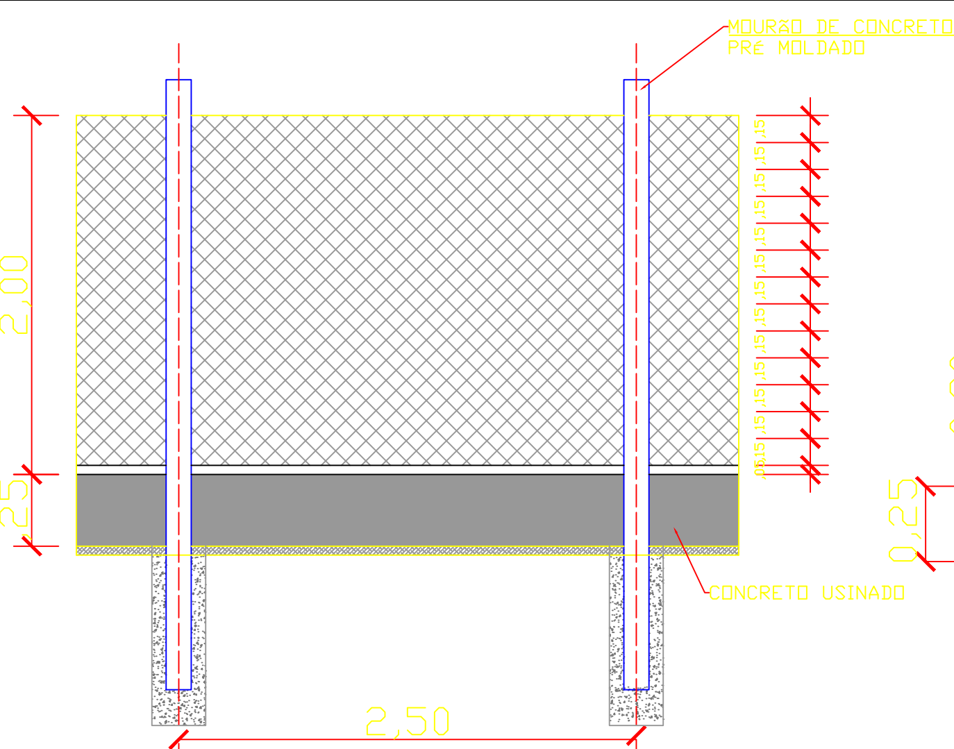
ELEVAÇÃO FRONTAL - Alambrado fechamento
