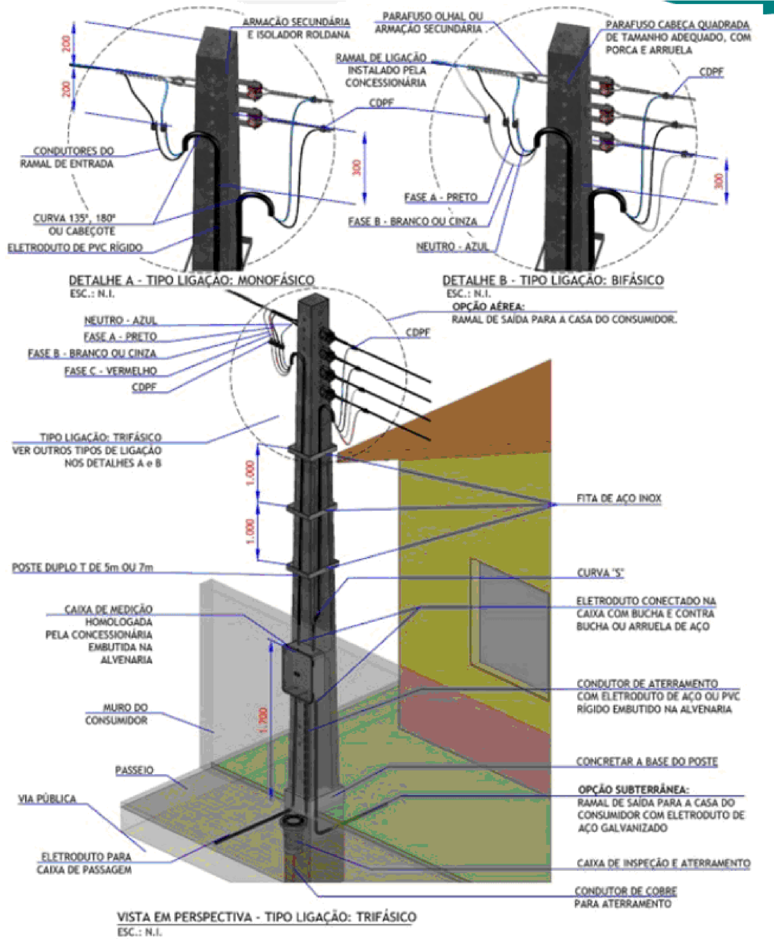
MODELO DE PADRÃO DE ENTRADA DE ACORDO COM A CONCESSIONÁRIA LOCAL
