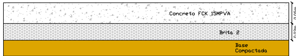
CORTE ESQ. (CALÇAMENTO) SEM ESCALA
