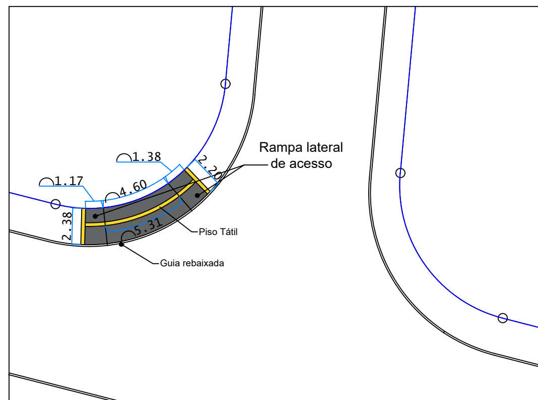
DETALHE 01 / RAMPA ACESSÍVEL ESC. 1:250
