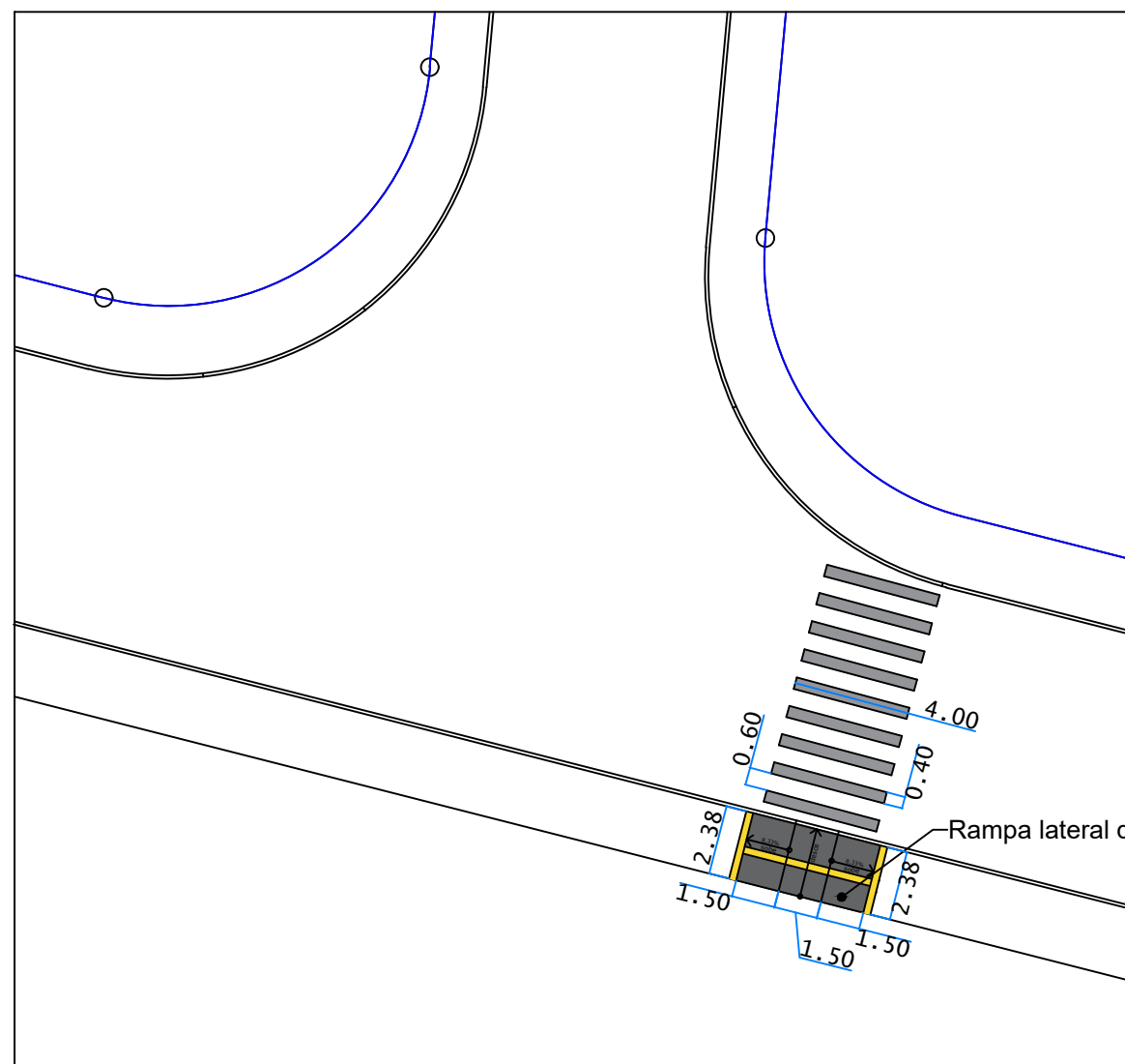
DETALHE 03 / FAIXA DE PEDESTRE + RAMPA ACESSÍVEL ESC. 1:250
