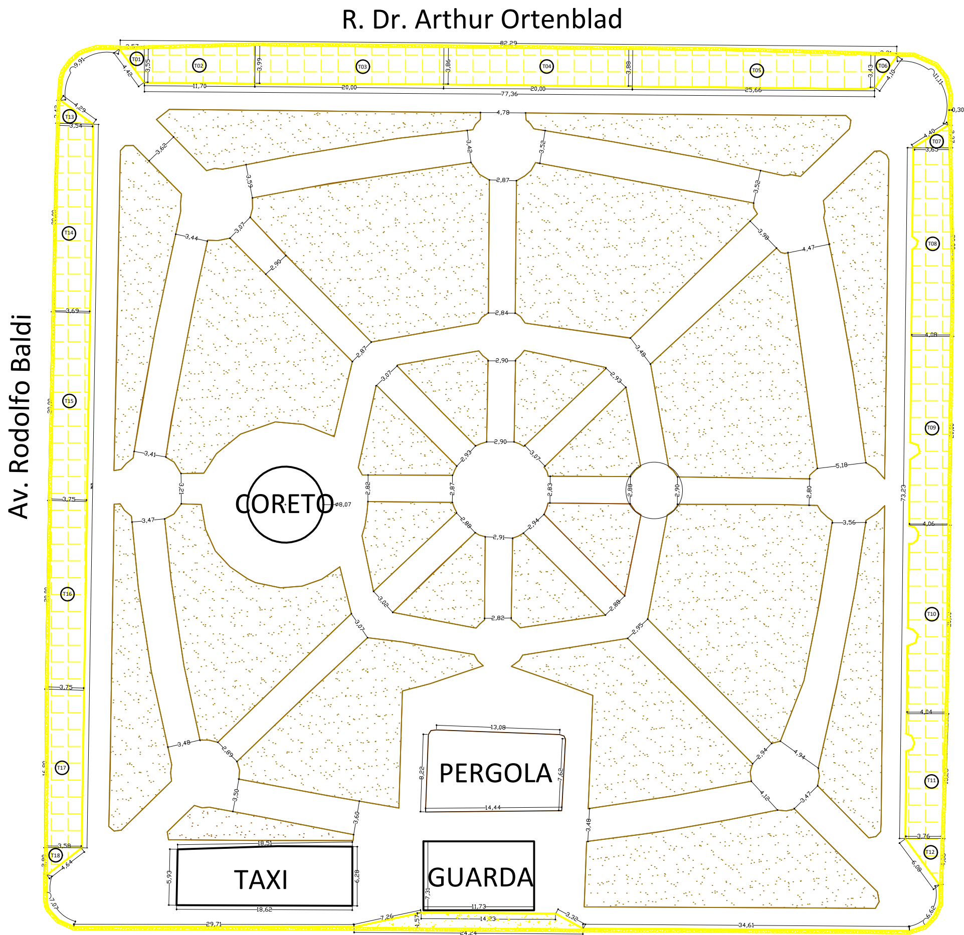
PLANTA DE DEMOLIÇÃO - ESTACIONAMENTO ESC. 1:400
