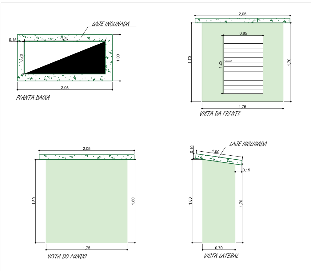
PADRÃO DE ENERGIA ESC. 1:50
