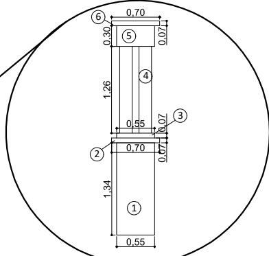
DETALHE DO PILAR
