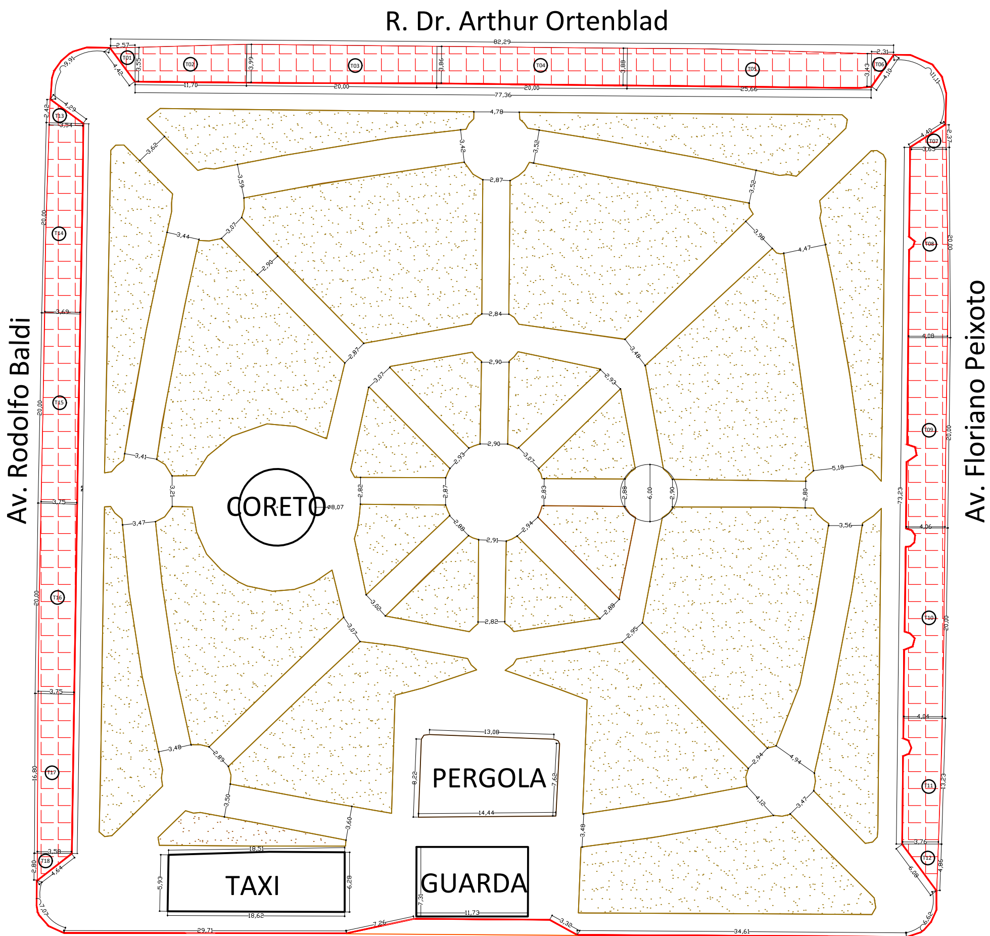
PLANTA DE RECOLOCAÇÃO PEDRA PORTUGUESA - ESTACIONAMENTO ESC. 1:400
