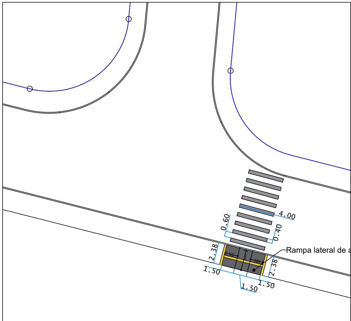
DETALHE 03 / FAIXA DE PEDESTRE + RAMPA ACESSÍVEL ESC. 1:250
