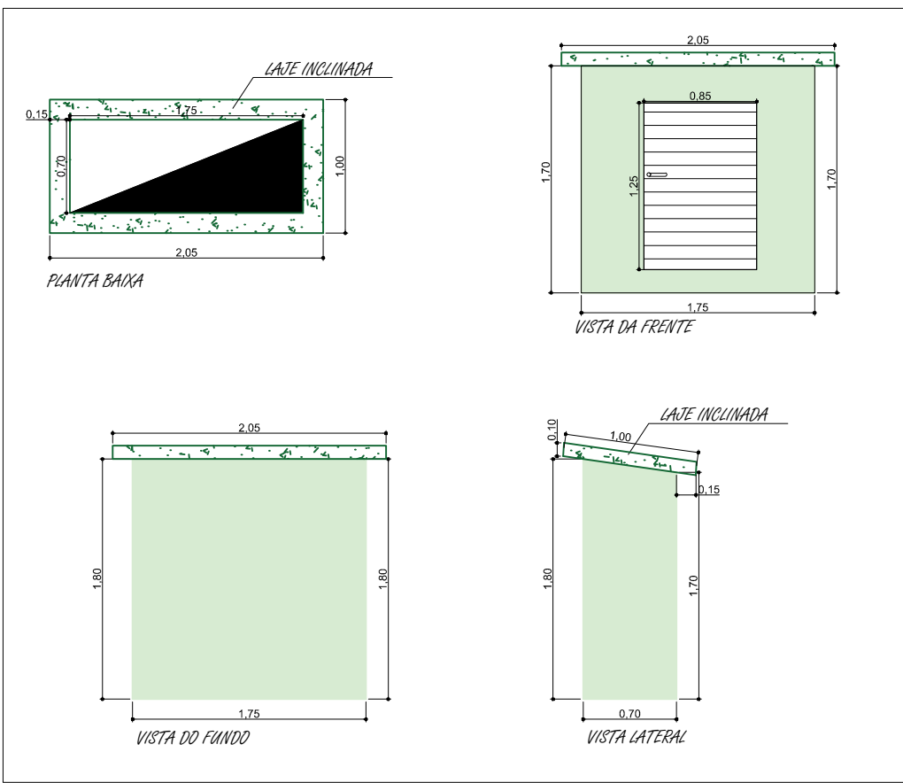
PADRÃO DE ENERGIA ESC. 1:50
