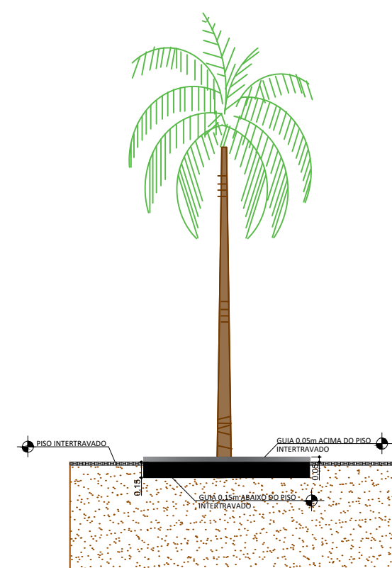
DETALHE REUTILIZAÇÃO DA GUIA
