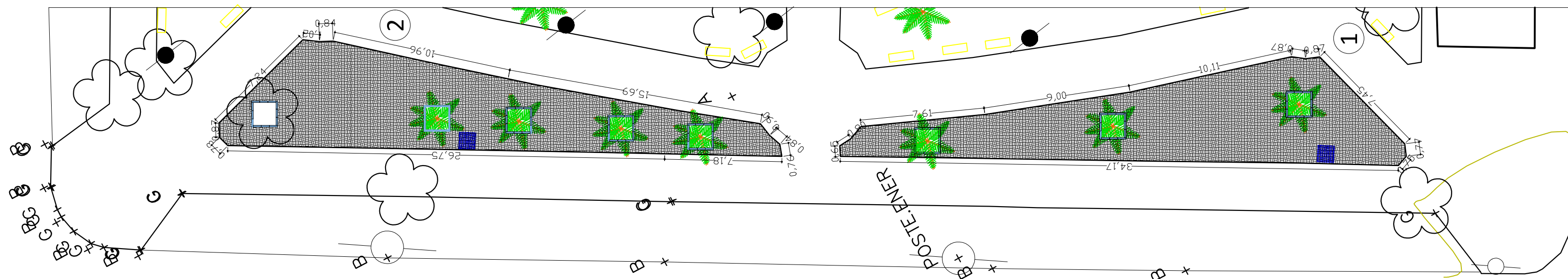
DETALHE REUTILIZAÇÃO DA GUIA
