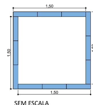
CANTEIRO PARA ÁRVORES
