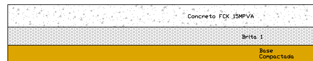
CORTE ESQ. (CALÇAMENTO) SEM ESCALA
