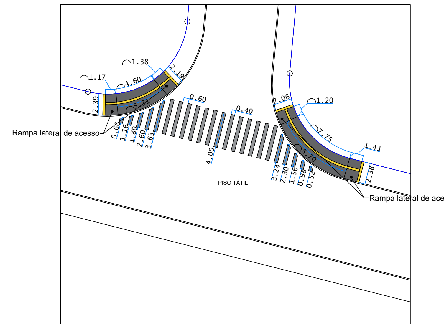
DETALHE 02 / FAIXA DE PEDESTRE + RAMPA ACESSÍVEL ESC. 1:250
