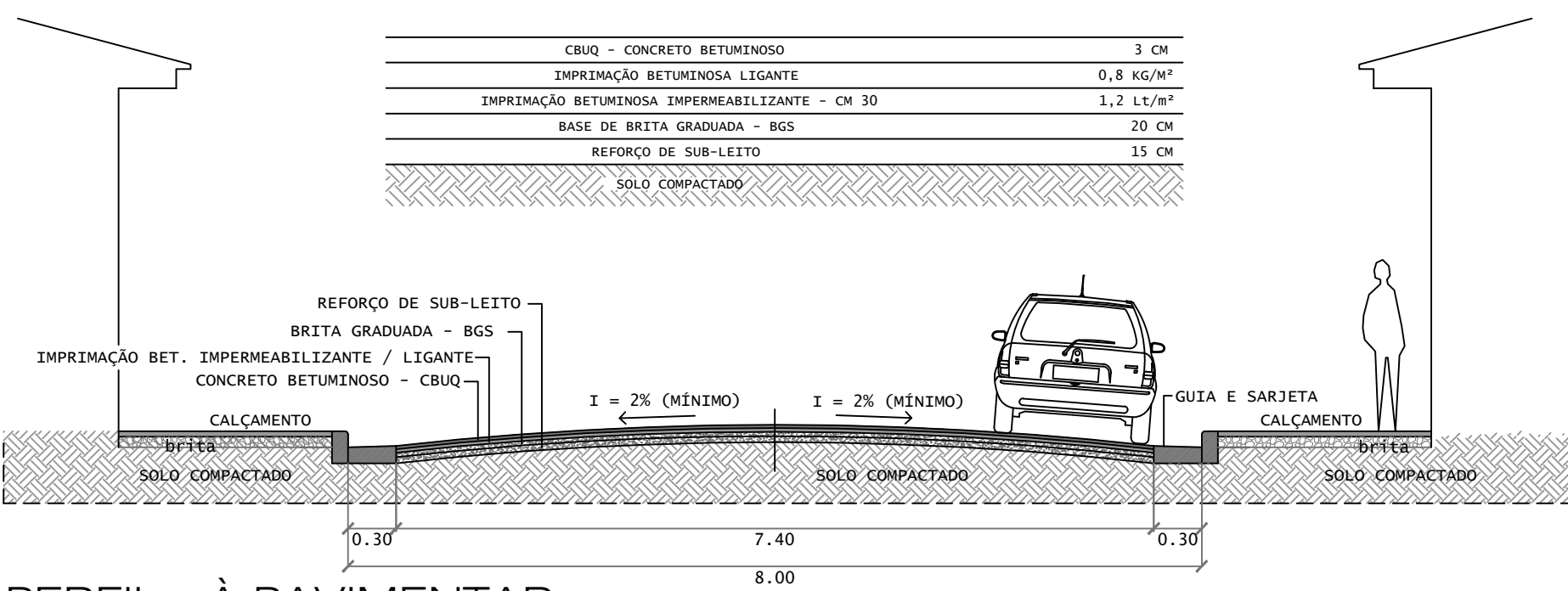
PERFIL - À PAVIMENTAR SEM ESCALA
