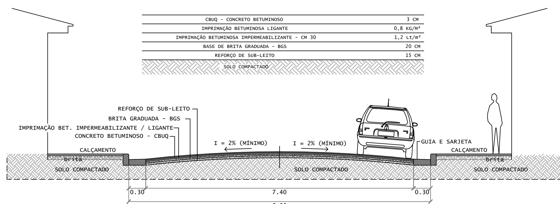
PERFIL - À PAVIMENTAR SEM ESCALA
