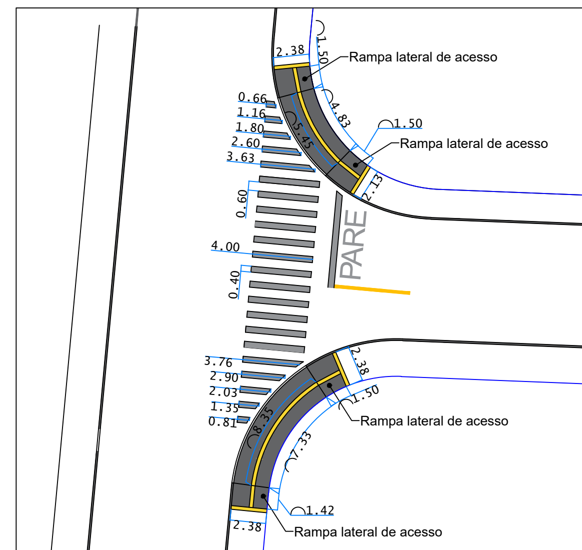
DETALHE 01 / FAIXA DE PEDESTRE + RAMPA ACESSÍVEL ESC. 1:250
